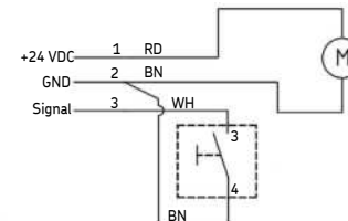
Schaltbild Leermeldesignal
