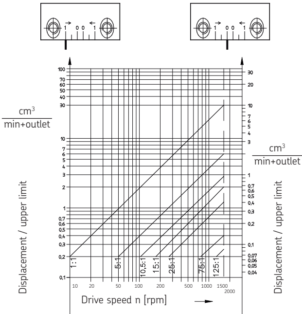
Fig. 2 Displacement
